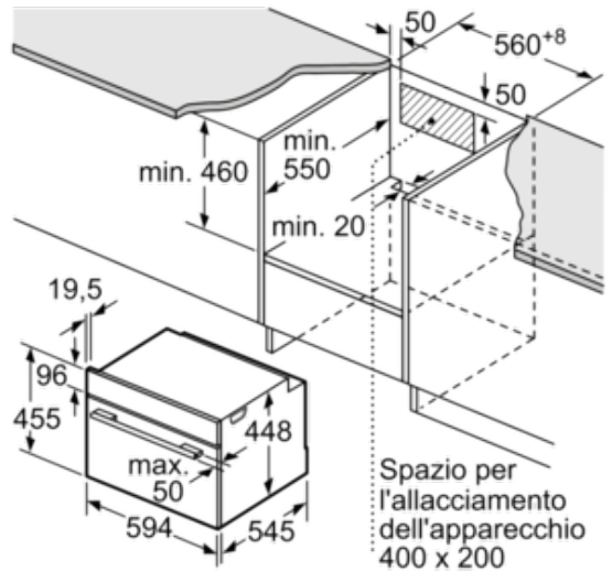
Spazio per l'allacciamento dell'apparecchio 400 x 200 Dimensioni in mm
